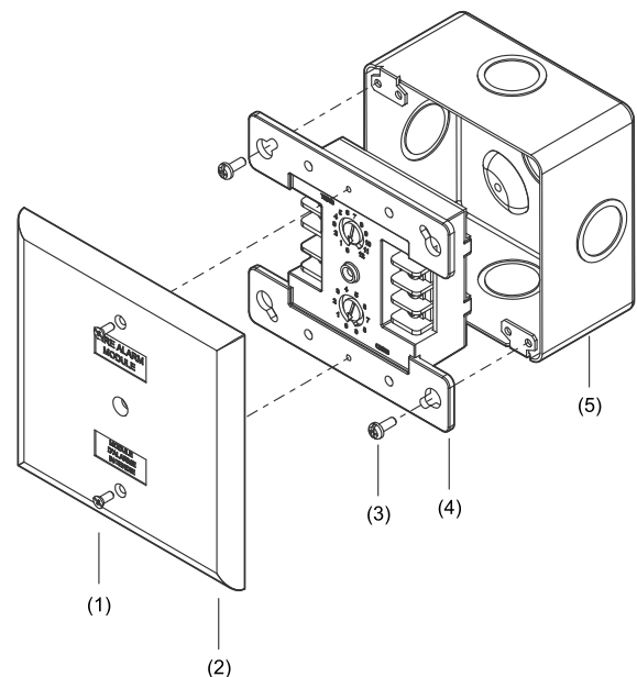
Figura 2: Instalación del módulo
