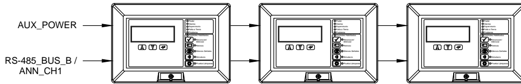
Figura 6: Cableado Clase B redundante Típico
