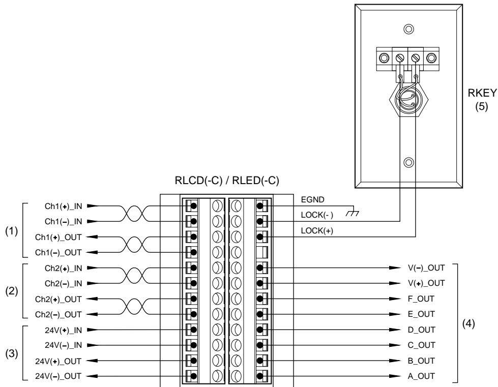
Figura 8: Cableado de anunciador típico
