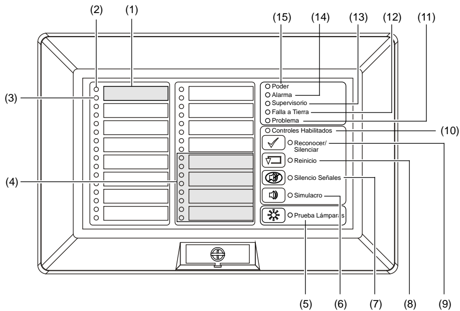
Figura 13: Controles e indicadores para RLED24 y RLED24R
