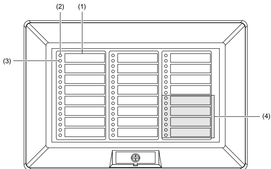
Figura 13: Controles e indicadores para RLED24 y RLED24R
